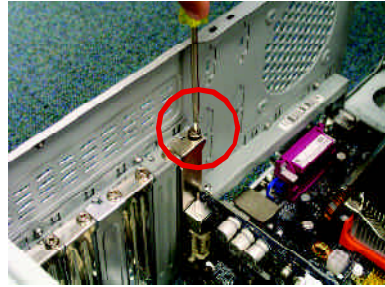
AGP 擴充槽
