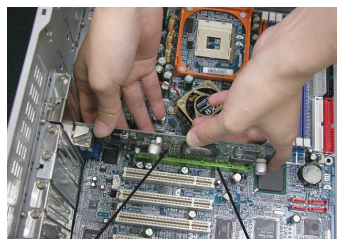
Графическая плата GV-R92S128T / GV-R92S64T Разъем AGP
