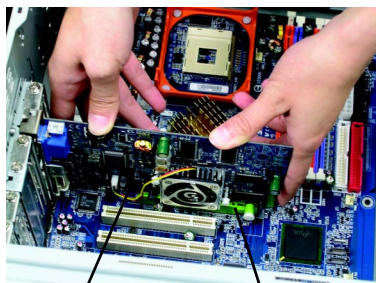
GV-R92128VH / GV-R92128DH / GV-R9264DHグラフィックス カード AGPスロット
