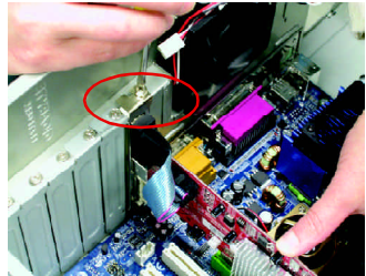
繪圖加速卡 AGP 擴充槽
