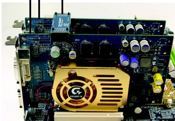
兩張相同型號的顯示卡 (例：GV-NX66T128D) SLI 連結器 (由主機板廠商提供)
