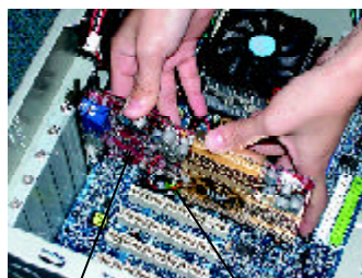
GV-R98P128D 繪圖加速卡 AGP 擴充槽
