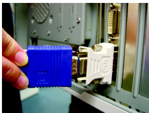
使用 DVI-I 轉 D-sub 轉接頭連接 VGA 螢幕
