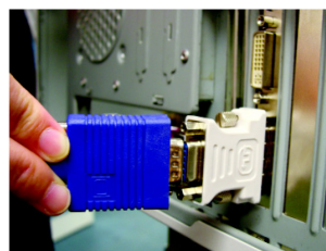
DVI-I-D-sub アダプタを経由して VGA モニタを接続します。
