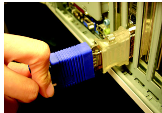
使用 DVI-I 轉 D-sub 轉接頭連接 VGA 螢幕
