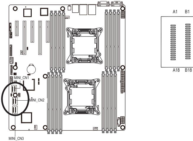
MINI_CN1
