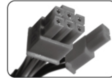
Connecteur PCI-E (6+2 broches)
