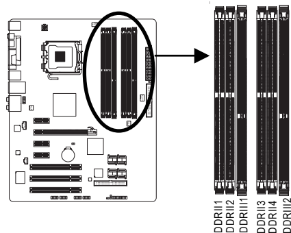
▶▶ DDR2 デュアルチャンネルメモリ構成表
