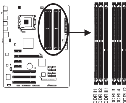
► DDR2 Bảng cấu hình bộ nhớ kênh kép
