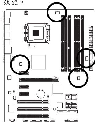
CPU_FAN (PCB rev. 2.0 之定義)：
