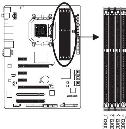
▶ デュアルチャンネルメモリ設定表
