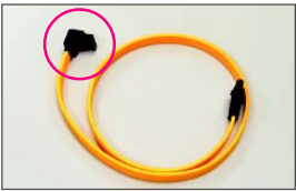
請將 SATA 3Gb/s 排線的 L 型接頭連接至 SATA 硬碟。
