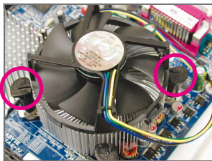
ขั้นที่ 3: วางตัวระบายความร้อนไว้บน CPU, จัดให้핀แบบผลึกทั้ง 4 ตรงกับรูพินบนเมนบอร์ด กดลงบน핀แบบผลึกในแนวทแยง
