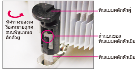
ขั้นที่ 2: ก่อนที่จะติดตั้งตัวระบายความร้อน, ให้สังเกตทิศทางของเครื่องหมายลูกศร บนพื้นแบบผลึกตัวผู้ (การหมุน พื้นแบบผลึกไปตามทิศทางของลูกศร จะเป็นการถอดตัวระบายความร้อนออก ถ้าหมุนในทางตรงข้าม จะเป็นการติดตั้ง)
