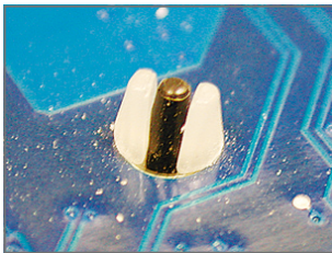
ขั้นที่ 5: หลังจากการติดตั้ง ตรวจสอบที่ด้านหลังของเมนบอร์ด ถ้า핀 แบบผลึกถูกใส่เหมือนรูปที่แสดงด้านบน หมายความว่าติดตั้งนั้นสมบูรณ์
