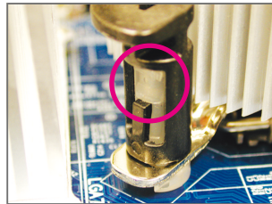
ขั้นที่ 4: คุณควรได้ยินเสียง “คลิก” เมื่อกดที่พื้นแบบผลึกแต่ละตัว ตรวจสอบว่า พื้นแบบผลึกตัวผู้และตัวเมียนั้นเชื่อมติดกัน (อ่านคู่มือการติดตั้งตัวระบายความร้อน CPU ของคุณ สำหรับขั้นตอนในการติดตั้งตัว ระบายความร้อน)
