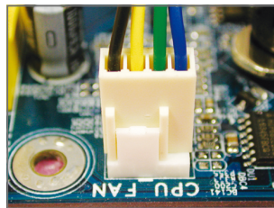
ขั้นที่ 6: สุดท้าย ให้เสียบขั้วต่อเพาเวอร์ของตัวระบาย ความร้อน CPU ไปยังหัวเสียบพัดลม CPU (CPU_FAN) บนเมนบอร์ด
