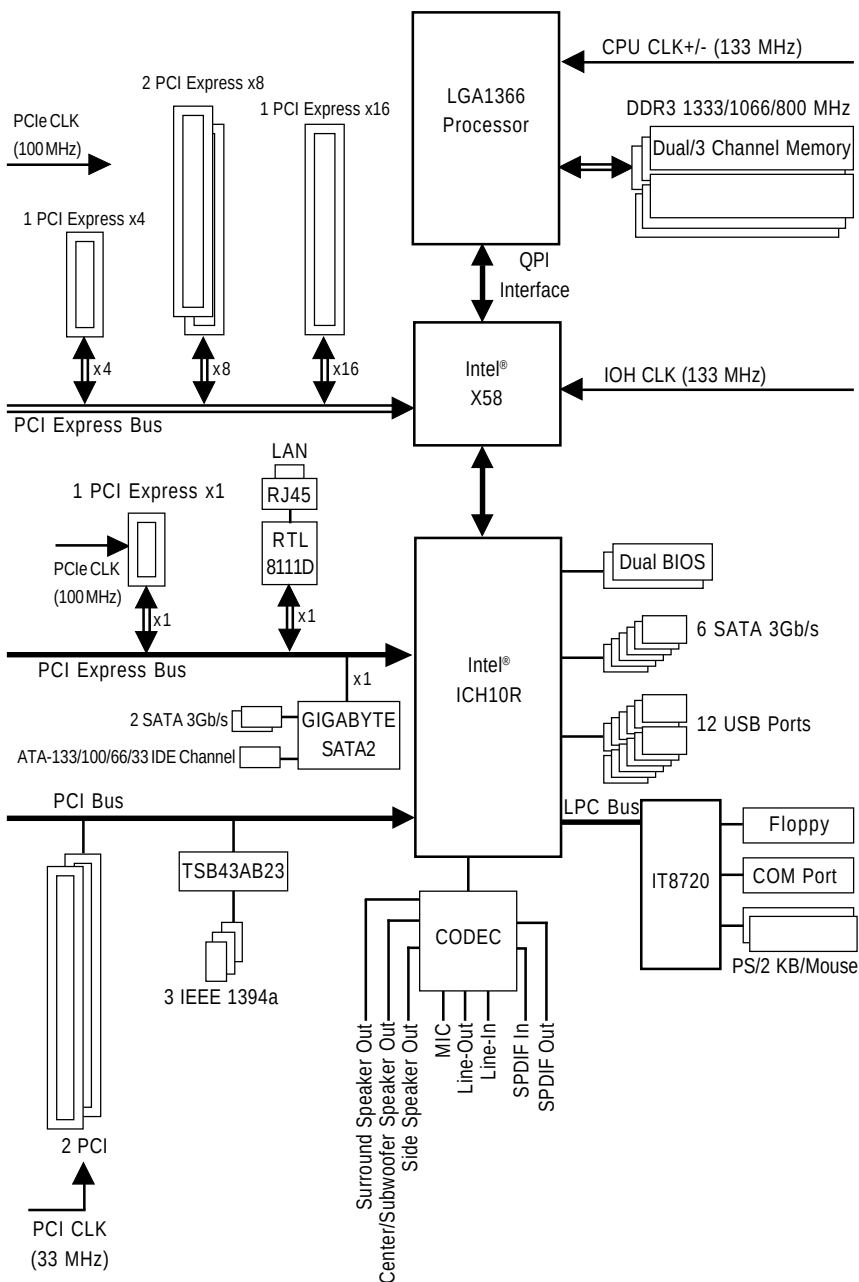
晶片組功能方塊圖
