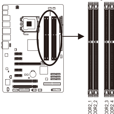
▶ デュアルチャンネルメモリ構成表
