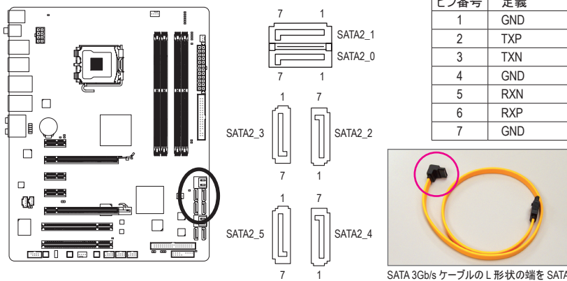
SATA 3Gb/s ケーブルの L 形状の端を SATA ハードドライブに接続してください。
