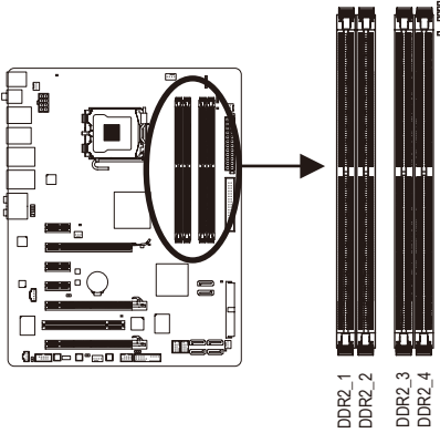
► Çift Kanallı Bellek Yapılandırma Tablosu
