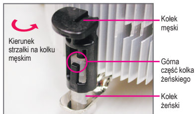
Rys. 2: Przed instalacją sprawdź, czy kierunek strzałki na kołku męskim nie jest skierowany do wewnątrz. Obróć kolek w kierunku wskazywanym przez strzałki, aby odłączyć zaczepy wentylatora. Obrócenie kołka w przeciwną stronę powoduje jego zamknięcie.
