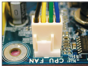
Rys. 6: Na koniec, podłącz przewód zasilania wentylatora do złącza wentylatora procesora na płycie głównej.
