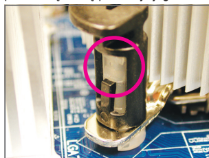
Rys. 4: Przy dociskaniu każdego z kołków powinieneś usłyszeć „kliknięcie”. Upewnij się, że kołki męski i żeński są prawidłowo połączone (szczegółowe informacje na temat instalacji zawarte są w instrukcji dołączonej do wentylatora).
