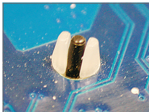
Rys. 5: Po instalacji sprawdź drugą stronę płyty głównej. Jeśli po włożeniu kolek wygląda jak na tym zdjęciu, instalacja jest zakończona.
