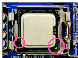
مرحله چهارم: پردازنده را میان انگشتان شصت و اشاره خود نگه دارید. پین شماره یک پردازنده را بیابید (با توجه به مثلث طلایی رنگ) و آن را با پین شماره یک بر روی سوکت پردازنده هم جهت کنید. (همچنین می‌توانید با استفاده از فرورفتگی‌های بر روی پردازنده و برآمدگی‌های بر روی سوکت، جهت صحیح قرار گیری آن را پیدا کنید.
