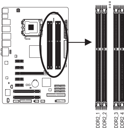
▶ 듀얼 채널 메모리 구성표
