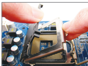
Fase 3: Rimuovere la protezione dalla piastra di carico. (Per proteggere la presa CPU, rimettere sempre il coperchio protettivo quando la CPU non è installata.)
