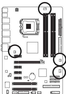
SYS_FAN1 / PWR_FAN
