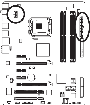
ATX_12V_2X
