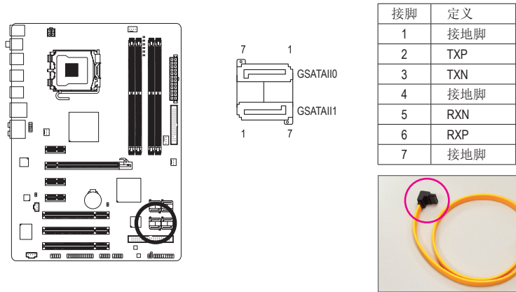
请将 SATA 3Gb/s 排线的 L 型接头连接至 SATA 硬盘。
