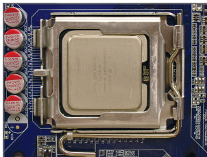
Fase 5: Una volta che la CPU è stata inserita in modo appropriato, rimettere la piastra di carico e spingere la leva socket CPU rimettendola nella sua posizione di blocco.
