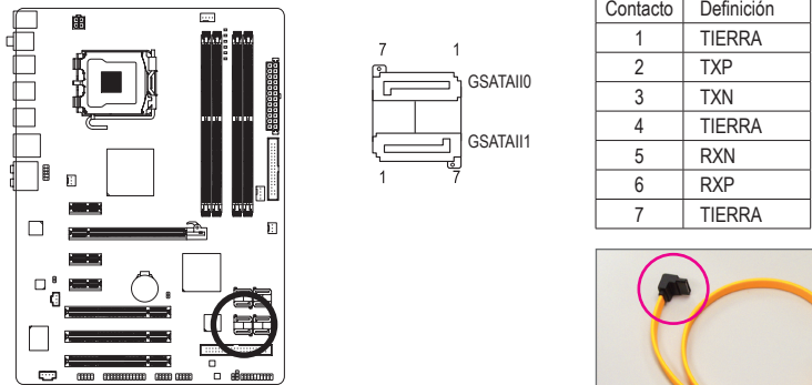
Conecte el extremo con forma de L del cable SATA de 3Gb/s a la unidad de disco duro SATA.
