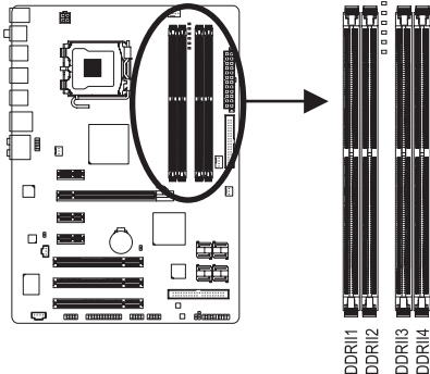
▶▶ Dualkanal-Speicherkonfigurationstabelle
