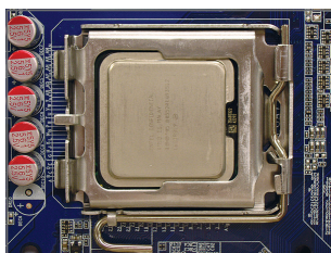
Fase 5: Una volta che la CPU è stata inserita in modo appropriato, rimettere la piastra di carico e spingere la leva socket CPU rimettendola nella sua posizione di blocco.
