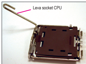
Fase 1: Sollevare completamente la leva socket CPU.
