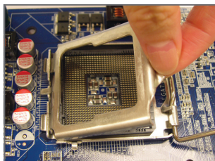
Fase 3: Sollevare la piastra di carico metallica sul socket CPU.
