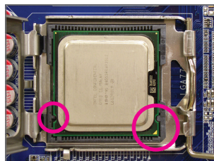
Fase 4: Tenere la CPU tra il pollice e l'indice. Allineare la marcatura Pin UNO della CPU (triangolo) con l'angolo Pin UNO del socket CPU (oppure allineare le dentellature della CPU con le tacche del socket) ed inserire delicatamente la CPU in posizione.
