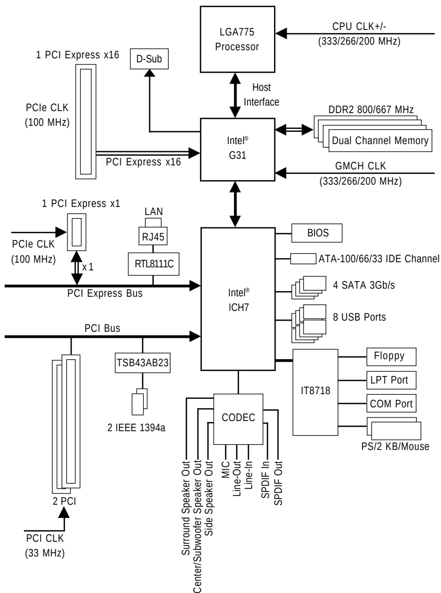
晶片組功能方塊圖
