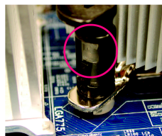
그림 4 수압 누름 핀들이 잘 조여졌는지 확인하십시오. (더 자세한 설치 지침은 사용자 매뉴얼의 방열판 설치 페이지를 참조하십시오)
