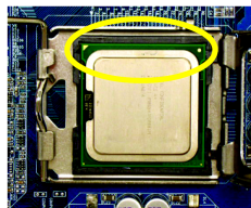
그림 3 CPU 소켓의 가장자리에 있는 작은 금색상각형을 주의하십시오. CPU 의 들어간 모서리를 삼각형에
