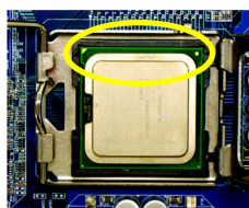
Abb. 3 Beachten Sie das kleine goldene Dreieck an der Kante der CPU-Fassung. Richten Sie die eingekerbte Ecke
