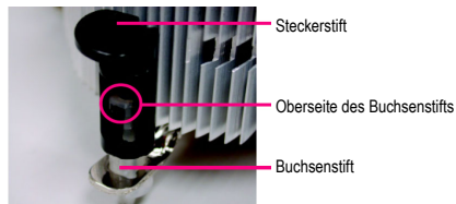
Abb. 2 (Zum Entfernen des CPU-Kühlers den Steckerstift in Pfeilrichtung drehen. Zum Installieren diesen Steckerstift in die entgegengesetzte Richtung drehen.) Beachten Sie, daß das Pfeilsymbol auf dem Steckerstift vor der Installation nicht nach innen zeigen darf. (Diese Anweisung gilt nur für Intel-Lüfter.)
