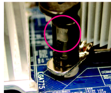
그림 4 수압 누름 핀들이 잘 조여졌는지 확인하십시오. (더 자세한 설치 지침은 사용자 매뉴얼의 방열판 설치 페이지를 참조하십시오)
