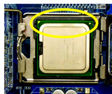
그림 3 CPU 소켓의 가장자리에 있는 작은 금색상각형을 주의하십시오. CPU 의 들어간 모서리를 삼각형에
