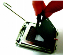
그림 2 CPU 소켓 위의 플라스틱 커버링을 제거하십시오.
