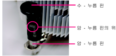
그림 2 (화살표 방향으로 누름 핀을 돌리면, CPU 방열판이 제거되고, 반대로 하면 설치됩니다.) 설치하기 전에 수 누름 핀에 표시된 화살표의 방향이 안쪽을 향하지 않는지 주의하십시오. (이 지침은 인텔 박스형 팬에만 적용됩니다)
