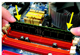
Abb. 1 Die DIMM Fassung hat eine Kerbe, so dass das DIMM Speichermodul nur in eine Richtung passen kann. Führen Sie das DIMM Speichermodul senkrecht in die DIMM Fassung ein. Dann drücken Sie es nach unten.
