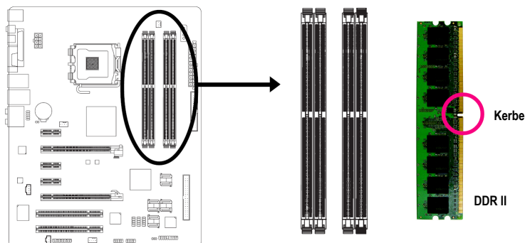
Abb. 1 Die DIMM Fassung hat eine Kerbe, so dass das DIMM Speichermodul nur in eine Richtung passen kann. Führen Sie das DIMM Speichermodul senkrecht in die DIMM Fassung ein. Dann drücken Sie es nach unten.
