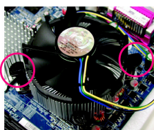
Abb. 3 Legen Sie den CPU-Kühler oben auf die CPU und stellen Sie sicher, dass die Steckerstifte nach dem Stiftloch der Motherboard ausgerichtet sind. Danach die Steckerstifte diagonal niederdrücken.
