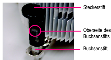
Abb. 2 (Zum Entfernen des CPU-Kühlers den Steckerstift in Pfeilrichtung drehen. Zum Installieren diesen Steckerstift in die entgegengesetzte Richtung drehen.) Beachten Sie, daß das Pfeilsymbol auf dem Steckerstift vor der Installation nicht nach innen zeigen darf. (Diese Anweisung gilt nur für Intel-Lüfter.)
