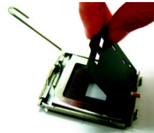
그림 2 CPU 소켓 위의 플라스틱 커버링을 제거하십시오.
