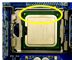
그림 3 CPU 소켓의 가장자리에 있는 작은 금속상각형을 주의하십시오. CPU 의들어간모서 리를 상각형에
