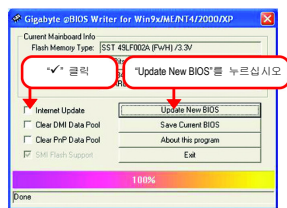
그림 3. @BIOS 유틸리티
