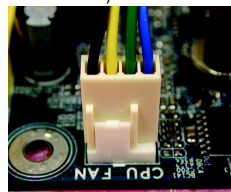
Figura 6 Por último, acople el conector de alimentación del disipador del microprocesador en la base de conexiones del ventilador del microprocesador que se encuentra en la placa base.
