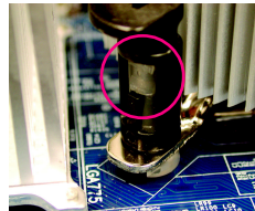
Figura 4 Asegúrese de que la chincheta macho y hembra están firmemente unidas. (Para obtener instrucciones detalladas sobre la instalación, consulte la sección de instalación del disipador del microprocesador que aparece en el manual del usuario.)
