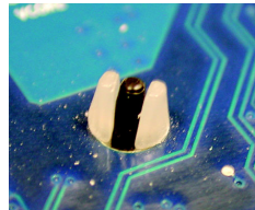
Figura 5 Compruebe la parte posterior de la placa base después de realizar la instalación. Si la chincheta está insertada como se indica en la figura, la instalación habrá terminado.
