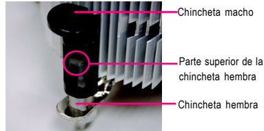
Figura 2 (Para retirar el disipador del microprocesador, gire la chincheta a lo largo de la dirección de la flecha. Gírela en sentido contrario para instalar el disipador.) Tenga en cuenta que la dirección de la flecha de la chincheta macho no está orientada hacia dentro antes de realizar la instalación. (Esta instrucción solamente se aplica al ventilador de Intel suministrado.)
