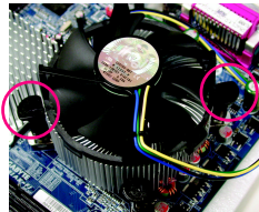
Figura 3 Coloque el disipador del microprocesador encima de éste y asegúrese de que las chinchetas apunten hacia el orificio situado en la placa base. Presione las chinchetas hacia abajo diagonalmente.
