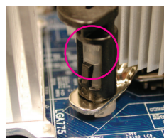
Рис. 4 Убедитесь, что штырек каждого крепежного элемента вошел в соответствующую гильзу. Подробная инструкция по установке приведена в разделе руководства, посвященном установке теплоотвода.
