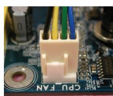
Рис. 6 Подключите штекер провода питания вентилятора теплоотвода к разъему CPU_FAN на системной плате. Установка завершена.
