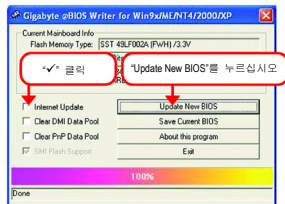
그림 3. @BIOS 유틸리티
