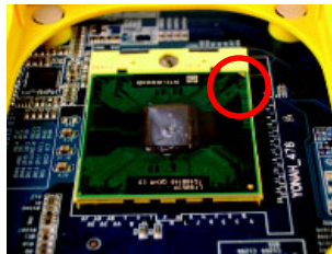
圖 2. 將中央處理器第一腳(金色三角形記號處)對齊插座上的缺腳記號，再將中央處理器小心放入插座中，並確定所有針腳都已進入插槽內。
