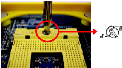
圖 1. 用一字螺絲起子將處理器插座上的螺絲設定在 🔓 位置。
