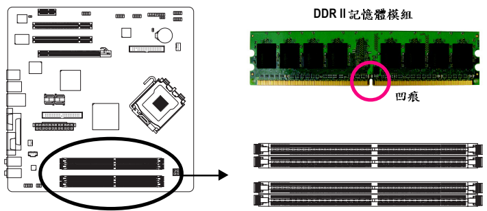
圖 1. 記憶體模組有一個凹痕，所以只能以一個方向插入。請扳開記憶體模組插槽卡榫，以雙手按在記憶體模組上邊兩側，以垂直向下平均施力的方式，將記憶體模組下壓推入插槽。
