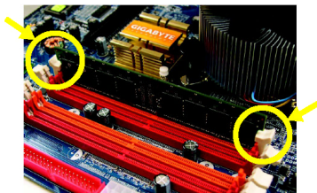
Fig. 2 Cierre el clip de plástico en ambos bordes del zócalo DIMM para enganchar el módulo DIMM. Invierta los pasos de instalación cuando quiera quitar el módulo DIMM.
