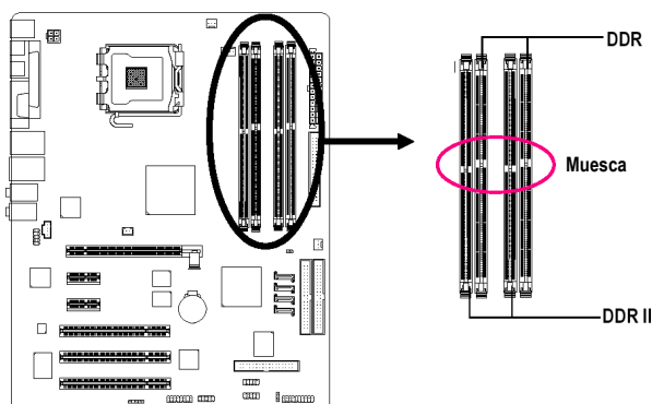
Fig. 1 El zócalo DIMM tiene una muesca, por lo tanto el módulo de memoria DIMM sólo puede encajar en una dirección. Insertar el módulo de memoria DIMM verticalmente en el zócalo DIMM. Después presiónelo hacia abajo.
