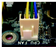
Fig. 6 Finalmente, por favor conecte el conector de alimentación del disipador al cabezal del ventilador de la CPU ubicado en la placa madre.
