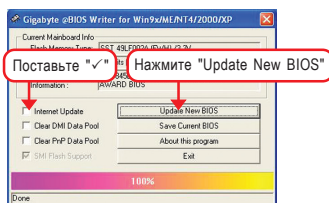
Рис. 3. Утилита @BIOS
