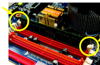
Fig. 2 Cierre el clip de plástico en ambos bordes del zócalo DIMM para enganchar el módulo DIMM. Invierta los pasos de instalación cuando quiera quitar el módulo DIMM.
