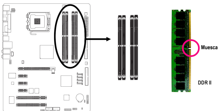
Fig. 1 El zócalo DIMM tiene una muesca, por lo tanto el módulo de memoria DIMM sólo puede encajar en una dirección. Insertar el módulo de memoria DIMM verticalmente en el zócalo DIMM. Después presiónelo hacia abajo.
