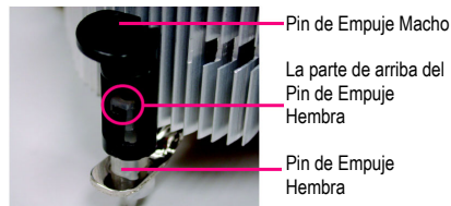
Fig. 2 (Se gira el pin de empuje en la dirección de la flecha para quitar el disipador, lo contrario es para instalar.) Por favor tenga en cuenta que la dirección de la flecha en el pin de empuje macho no mire hacia dentro antes de la instalación. (Estas instrucciones son sólo para ventiladores con caja Intel)
