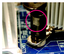
Fig. 4 Por favor asegúrese de que los pin Macho y Hembra están unidos conjuntamente. (Para instrucciones detalladas sobre la instalación, por favor consulte la sección de instalación del disipador del manual del usuario).
