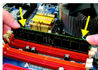
Fig. 1 El zócalo DIMM tiene una muesca, por lo tanto el módulo de memoria DIMM sólo puede encajar en una dirección. Insertar el módulo de memoria DIMM verticalmente en el zócalo DIMM. Después presiónelo hacia abajo.
