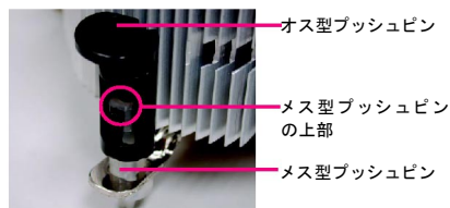
図 2 (プッシュピンを矢印方向に回し、ヒートシンクを取り外します。その反対は装着となります。)
