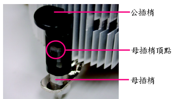
圖 2. 順著公插梢箭頭方向為移除散熱裝置；反之，安裝散熱裝置前請先將公插梢旋轉回原本位置。(此範例為 Intel 盒裝風扇)
