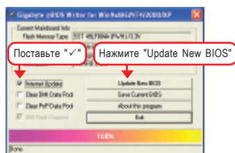
Рис. 3. Утилита @BIOS
