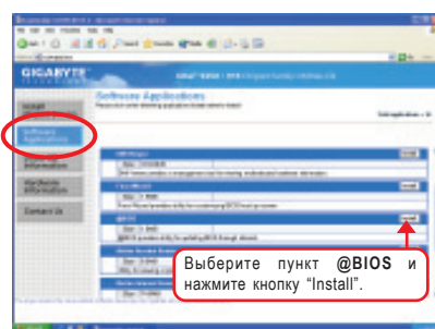
Рис. 3. Утилита @BIOS
