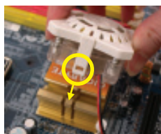
Рис. 1 Для установки вентилятора Cool-Plus на теплоотвод совместите выступы на двух противоположных сторонах вентилятора с выемками на краях теплоотвода (см. рис.) Нажмите на вентилятор,
