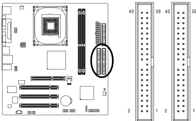
第二組 IDE 插座 第一組 IDE 插座
