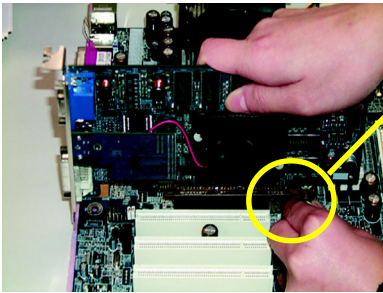
AGP 卡
